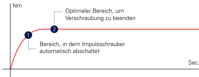
Beispiel einer harten Verschraubung
