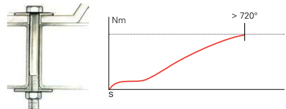
Beispiel einer weichen Verschraubung
