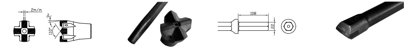
BOHRSTANGEN: BUCHSE 22 MM 6K X 108 MM FÜR HÄMMER: TOKU TJ-15LBS / TJ-20LBS
