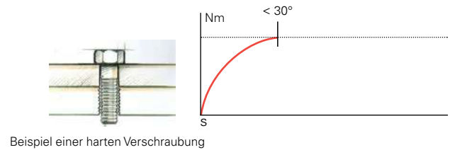
Beispiel einer harten Verschraubung
