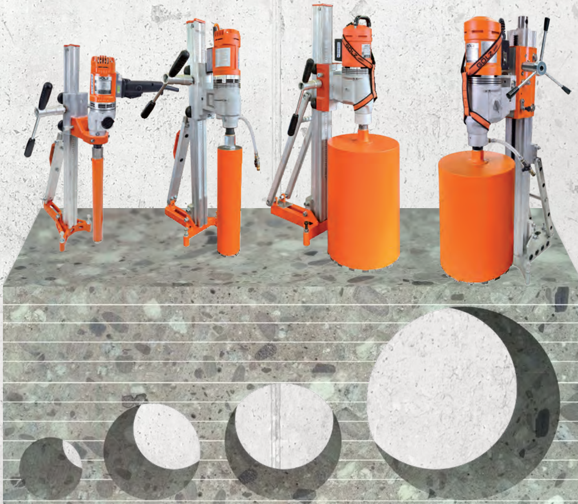
Ø 160 mm
