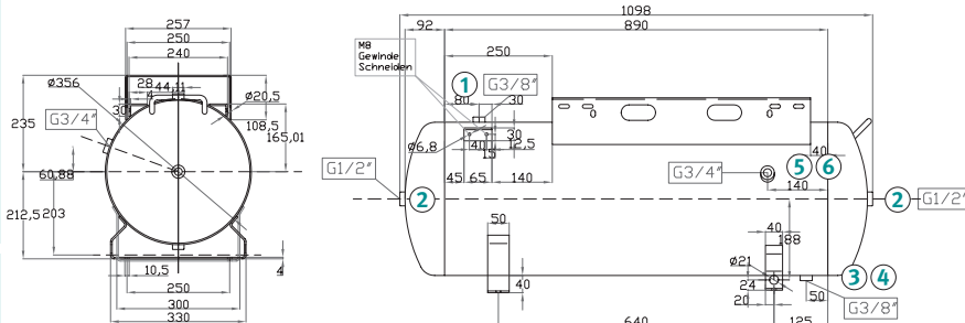
M ACDB 100/10 H MK mit Konsole ACDB 100/15 H MK verzinkt mit Konsole
